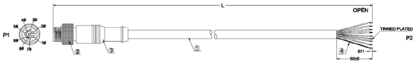
ケーブル外観図 : CAB-BVS-IO-1-XM
