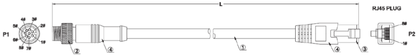
ケーブル外観図 : CAB-BVS-E-2-XM
