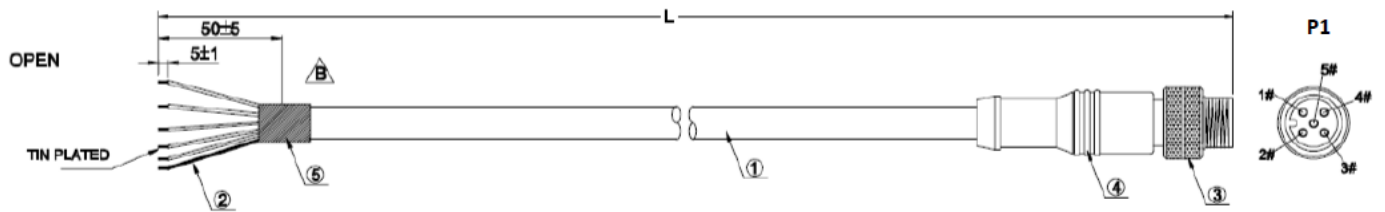
ケーブル外観図 : CAB-BVS-L-0-XM
